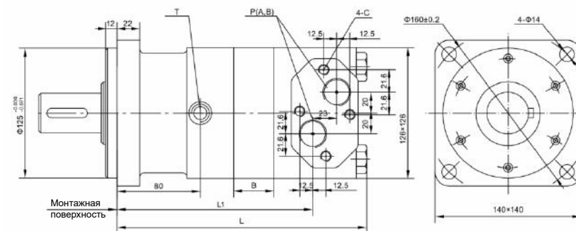
Квадратный фланец типа А
