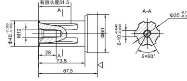
H5:φ40 прямоугольный шлицевой вал,6-40X35X10
