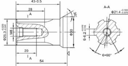
НЗ: ф30 прямоугольный шлицевой вал, 6-25,3-21,4-6,2
