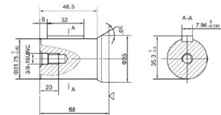
P5:Вал плоской шпонкиф31,75, плоская шпонка 7,96x7,96x32
