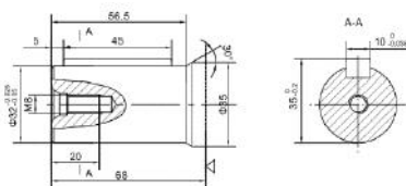
P6:Вал плоской шпонкиф32, плоская шпонка 10x8x45
