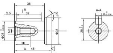
P4:Вал плоской шпонкиф25, плоская шпонка 8x7x32
